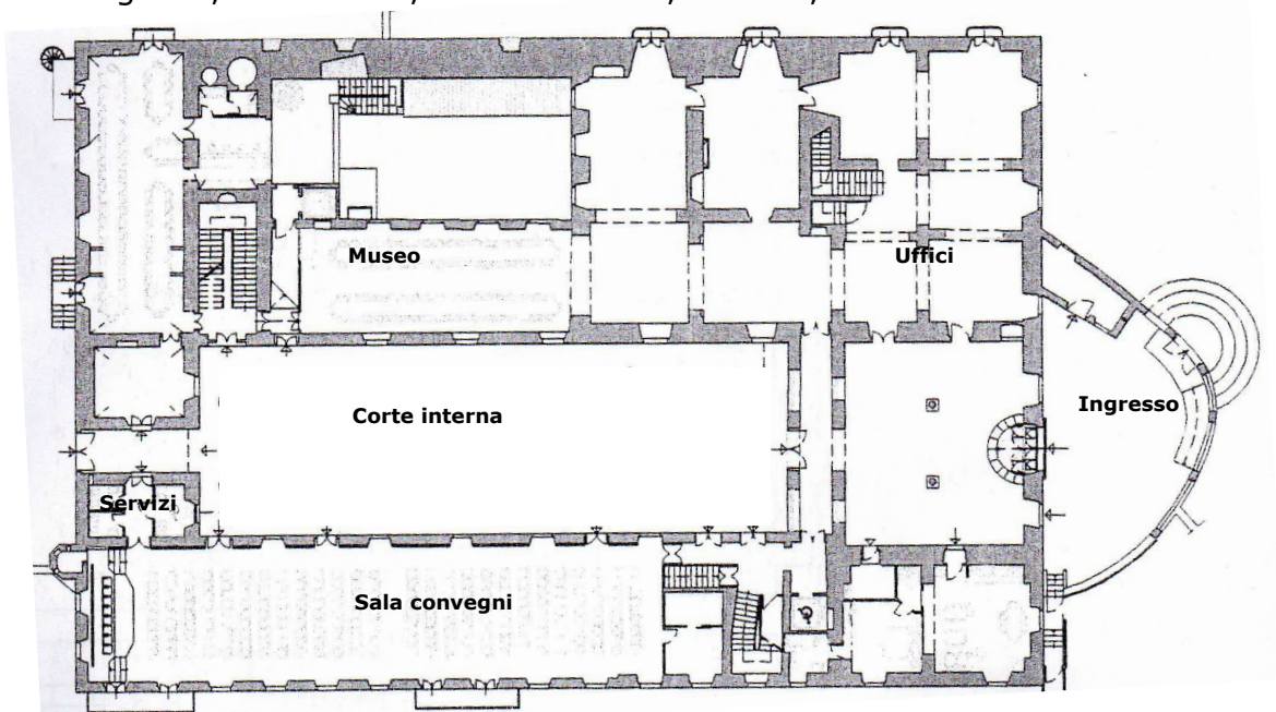
Fig. 1 Pianta del piano terra del Castello di Ladislao in gestione alla Fondazione Umberto Mastroianni
